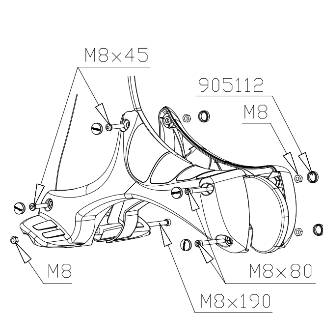
DET 5
