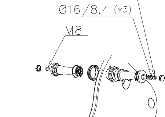
DET 3
